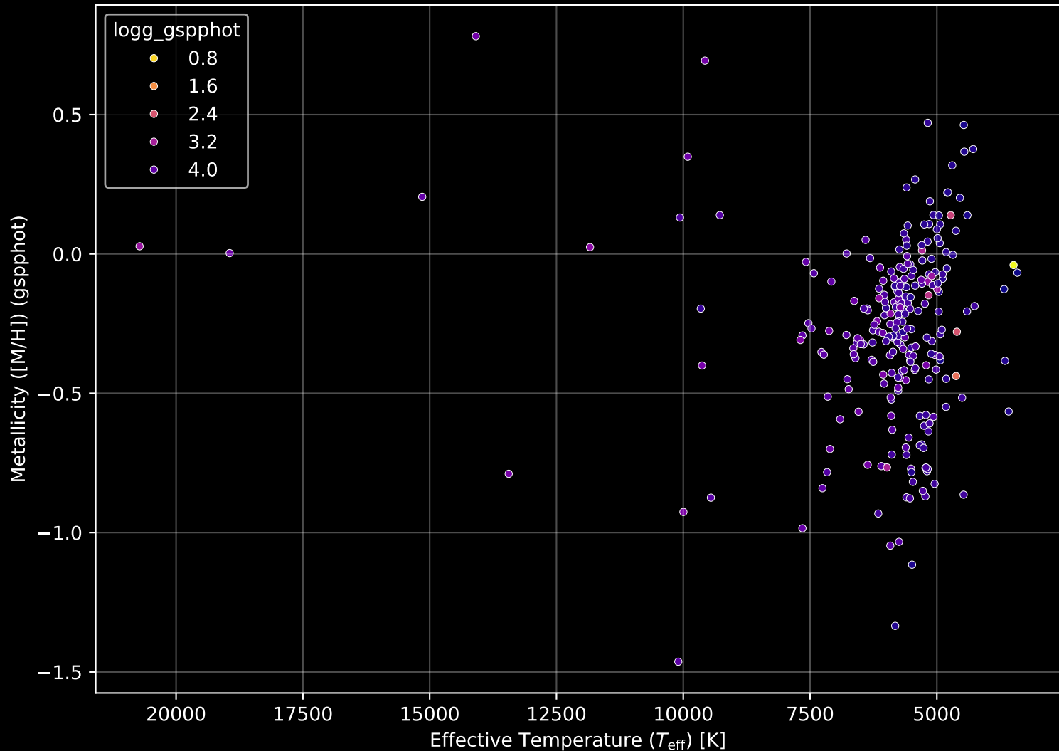
APOGEE DR17 Field: [K19_076+07_btx] Stellar Population Parameters (n= 252)
